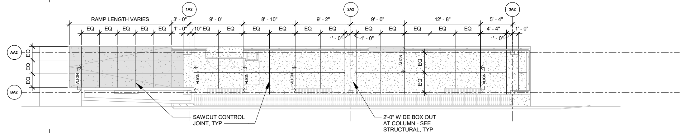
Scale: 1" = 10'-0"
