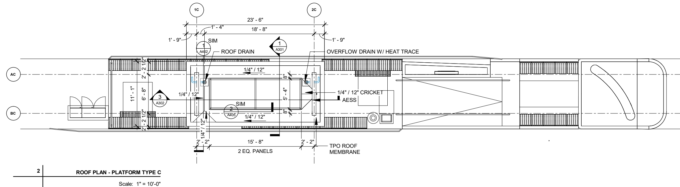
Scale: 1" = 10'-0"
